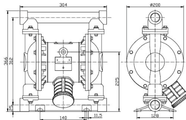
Монтажные отверстия
