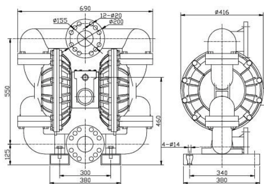
Монтажные отверстия
