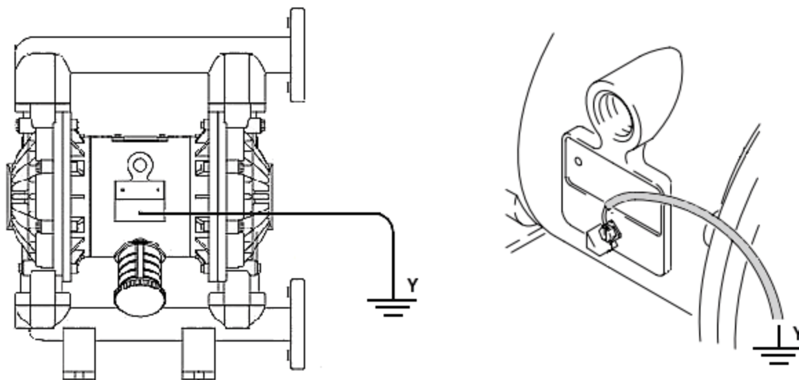
Рисунок 5. Заземление насоса
