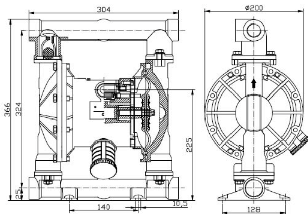
Монтажные отверстия
