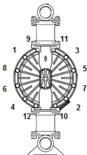
Рисунок 7. Очередность подтяжки болтовых соединений основных рабочих камер.
